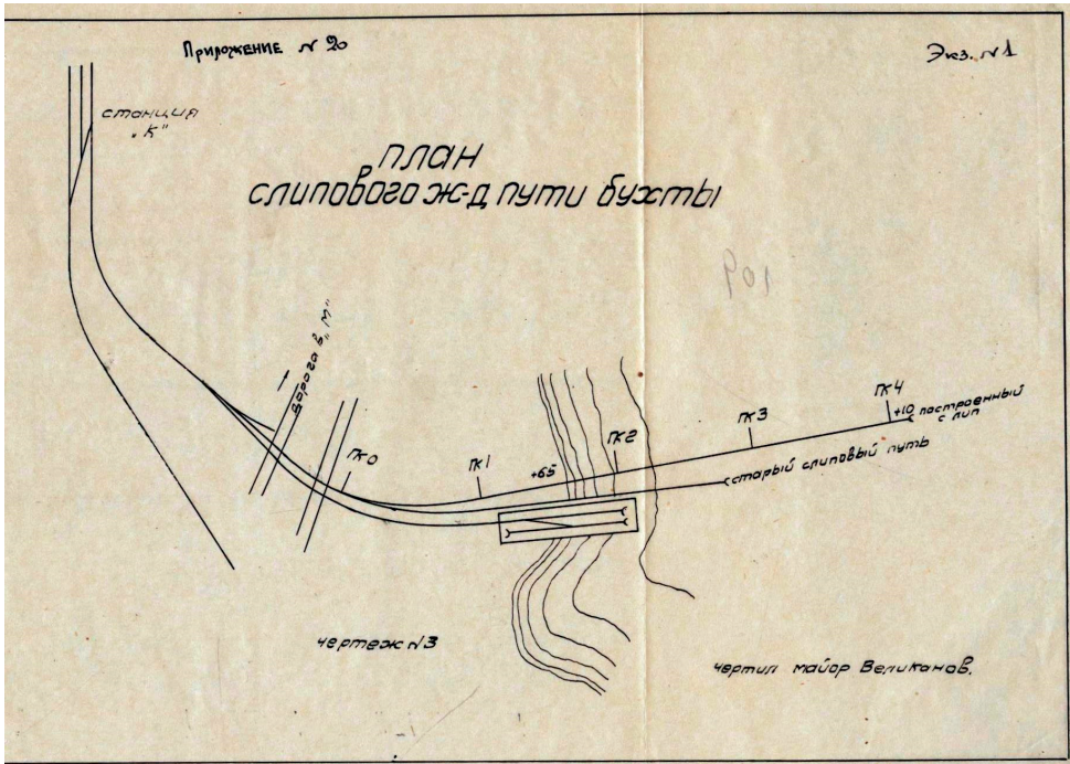
Рис. 4. План слипового железнодорожного пути для спуска подводных лодок в Ладожское озеро. Филиал ЦАМО РФ (архив ВМФ). Ф. 161. Оп. 33. Д. 17. Л. 109
