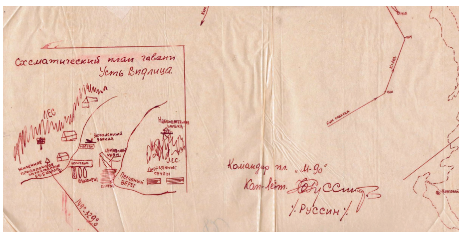
Рис. 10. Схематический план гавани Усть-Видлиця. Филиал ЦАМО РФ (архив ВМФ). Ф. 312. Оп. 3. Д. 1. Л. 82-3
