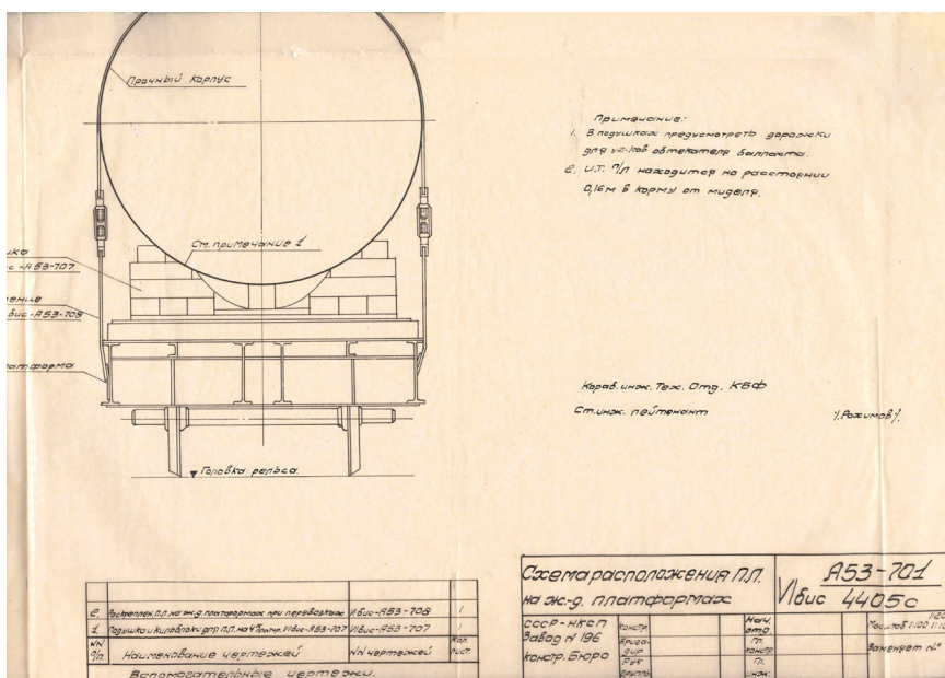
Рис. 3. Размещение подводной лодки на железнодорожной платформе. Филиал ЦАМО РФ (архив ВМФ). Ф. 161. Оп. 33. Д. 17. Л. 112. Ч. 1
